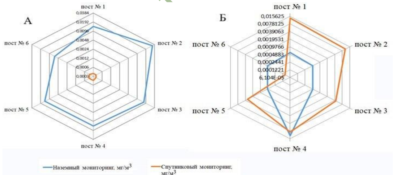
Рис. 2. Значения концентраций диоксида азота (а) и диоксида серы (б), полученные путём наземного и спутникового мониторинга (30.03.2025).
