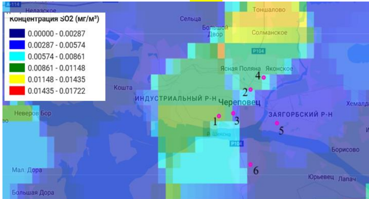
Рис. 1. Цифровая карта концентрации диоксида азота (а) и диоксида серы (б) по данным спутника Sentinel-5P в районе Череповца (30.04.2025). Точками обозначены станции наземного мониторинга: 1 — пост № 1 (район ДКС), 2 — пост № 2 (Привокзальный сквер), 3 — пост № 3 (стадион Metallurg), 4 — пост № 4 (район химико-технологического колледжа), 5 — пост № 5 (СОШ № 7), 6 — пост № 6 (аквапарк «Радужный»).
